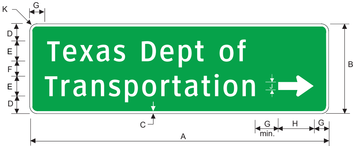
D26-10TR
