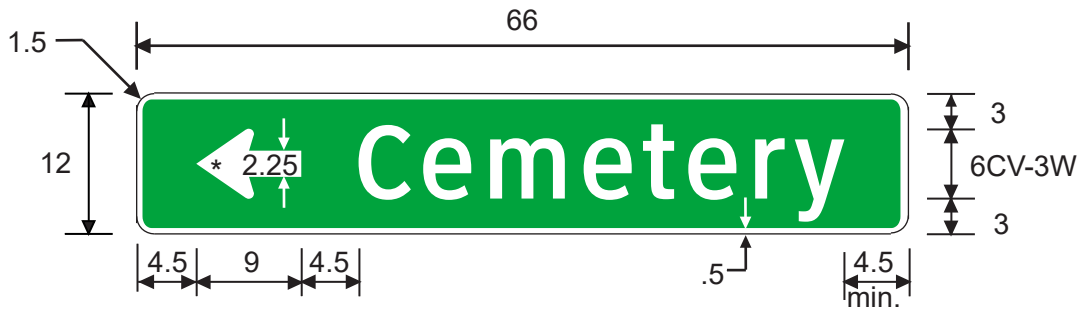
D3-3aTL
