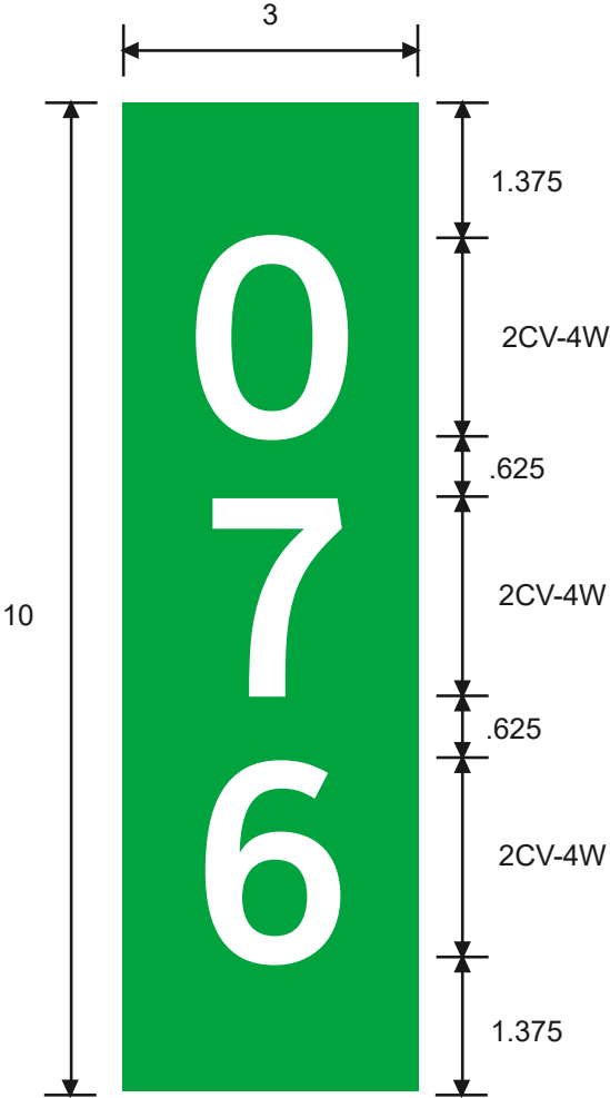
D10-7aT
