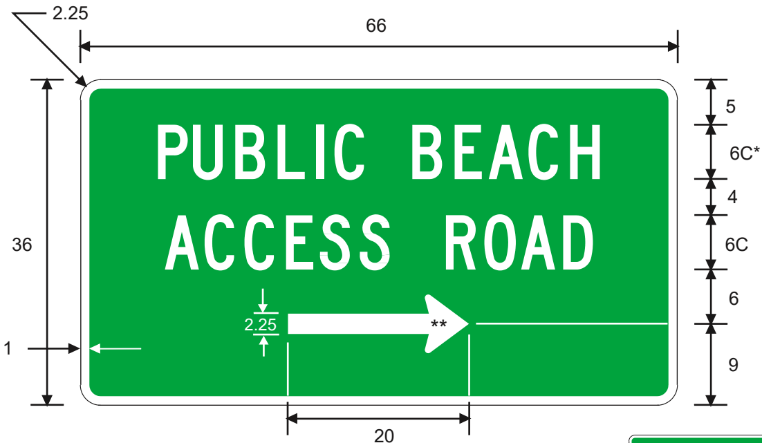
D24-2TR
