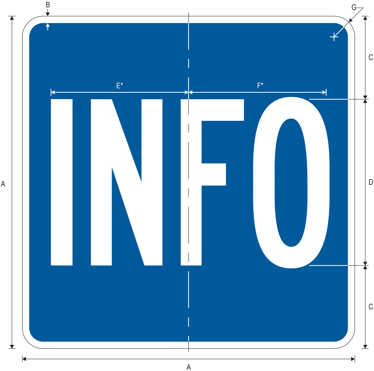
D9-10 INFO
