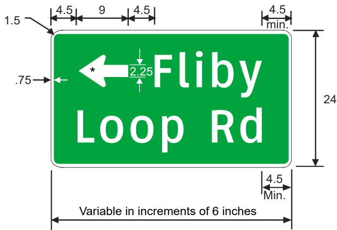
D21-1aT (L)
