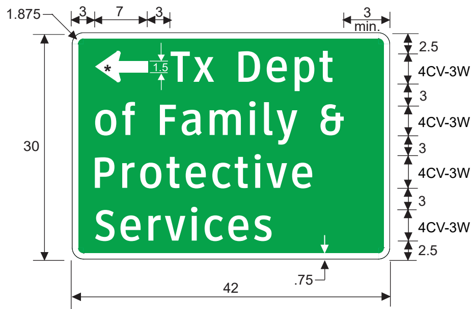
D26-5TL
