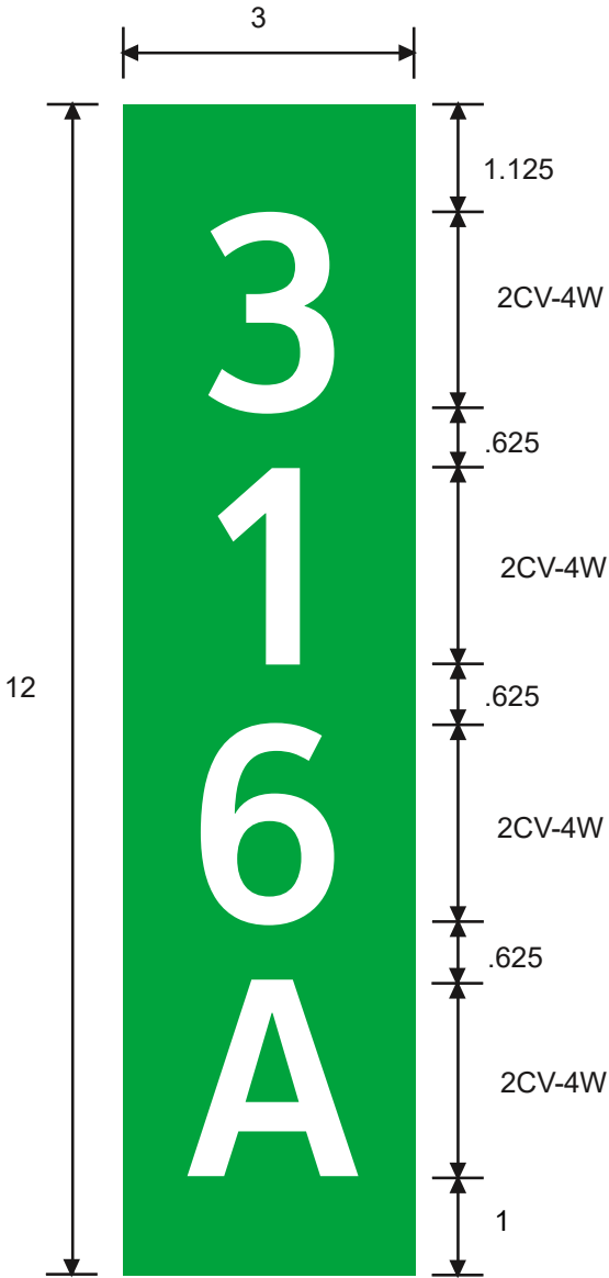
D10-7bT
