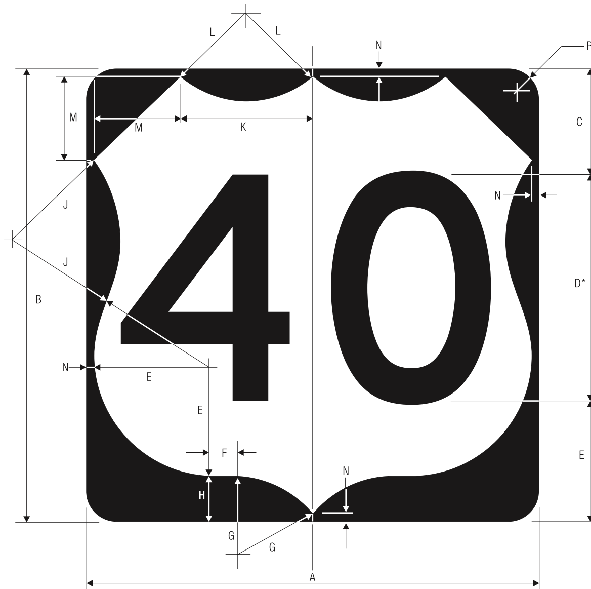
M1-4
