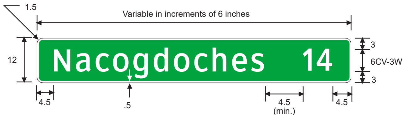
D2-1 Distance (1 line)
