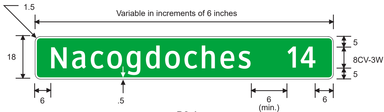
D2-1
