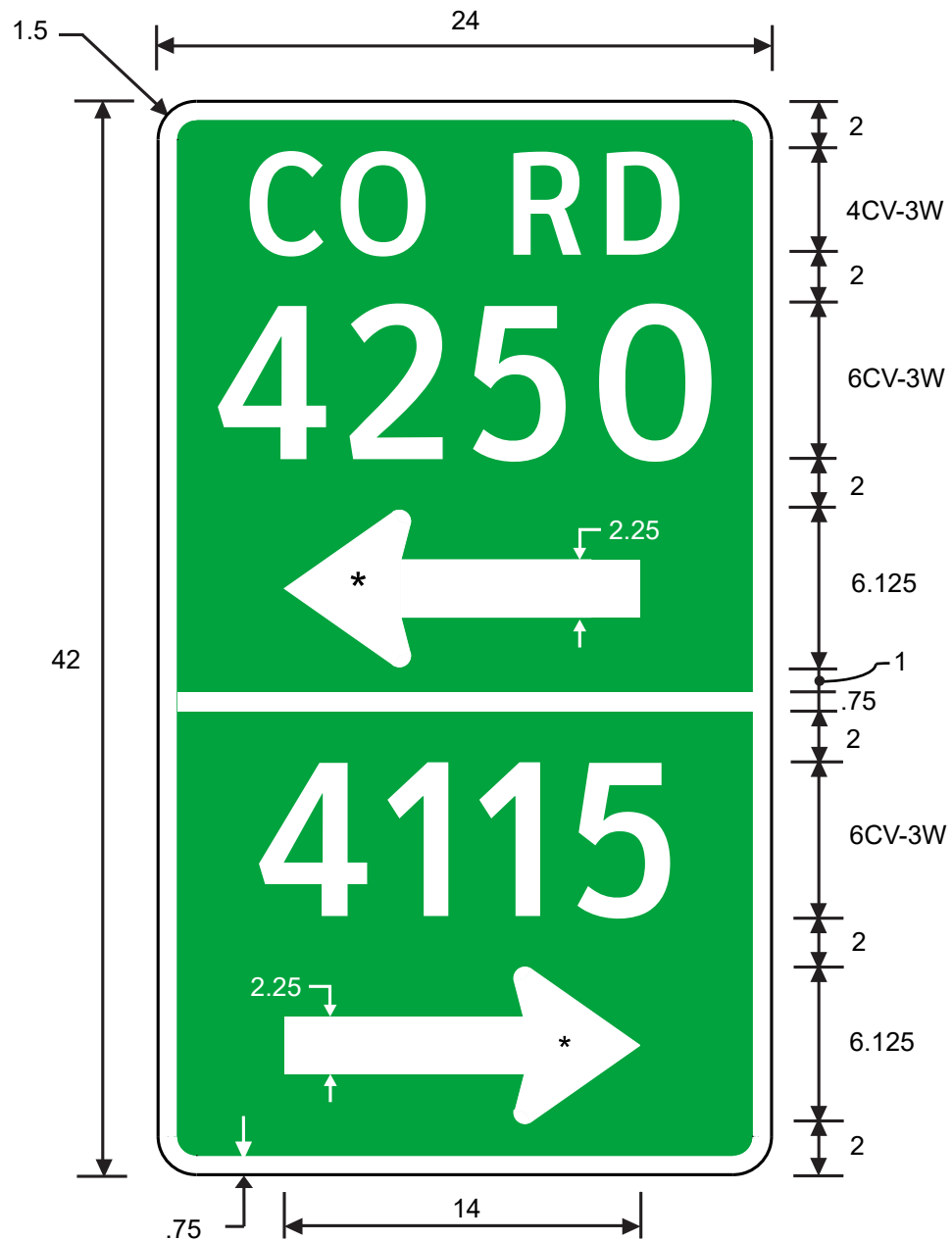
D20-5T (L, R) COUNTY ROAD
