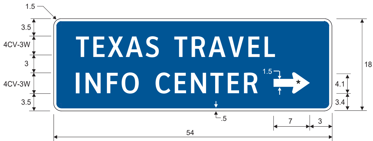
D12-5bTR
