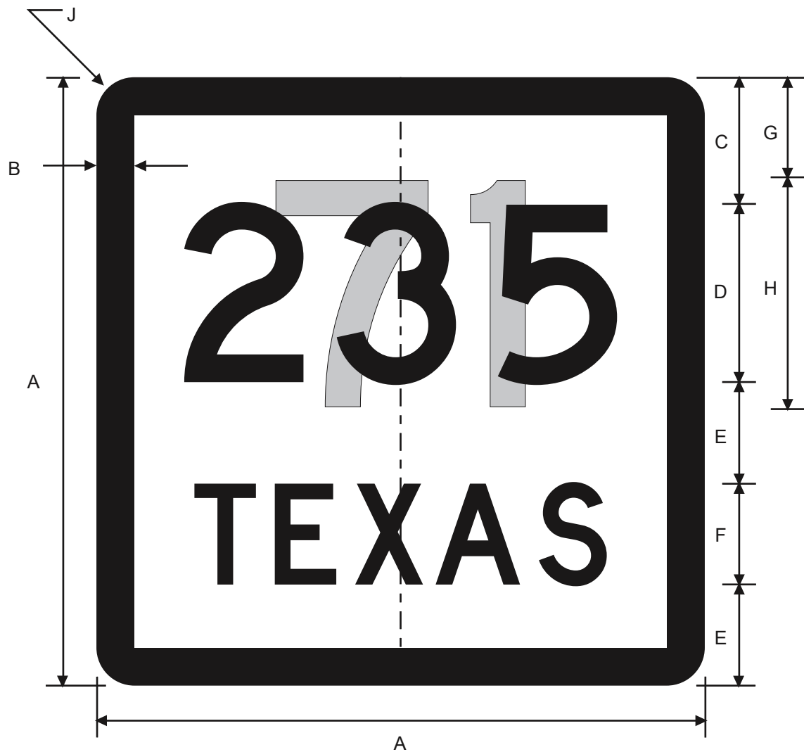
M1-6T
