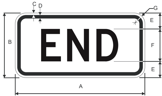
M4-6 END
