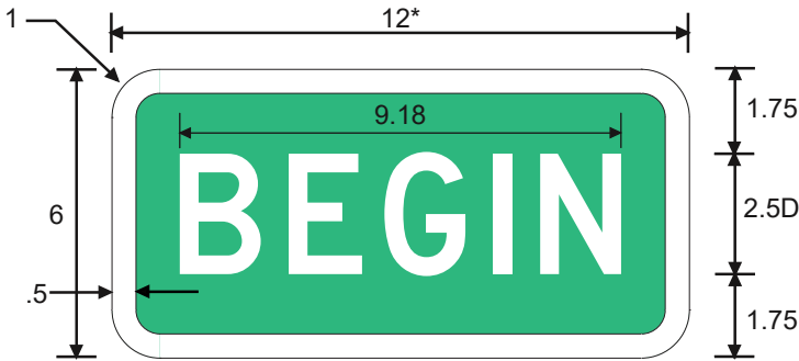
M4-14G
