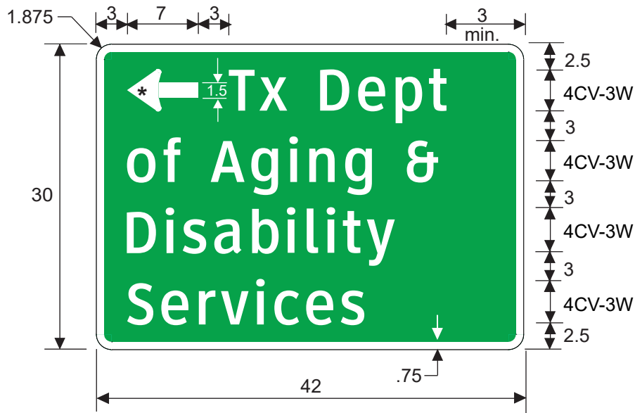
D26-4TL
