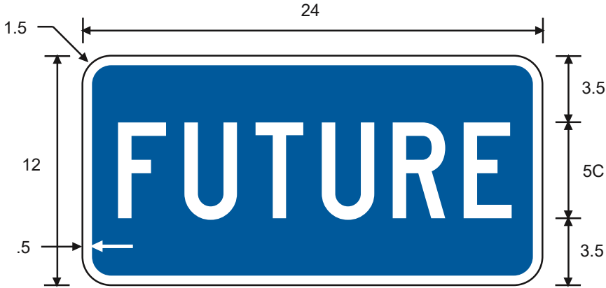
M4-7bT - FUTURE
