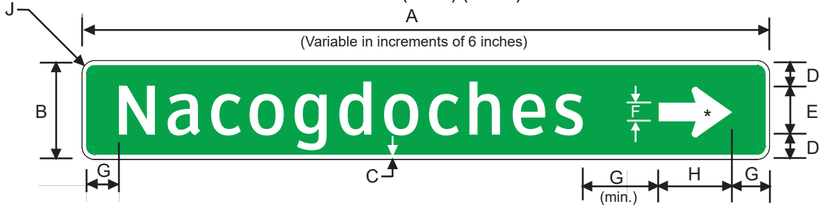
D1-1R
