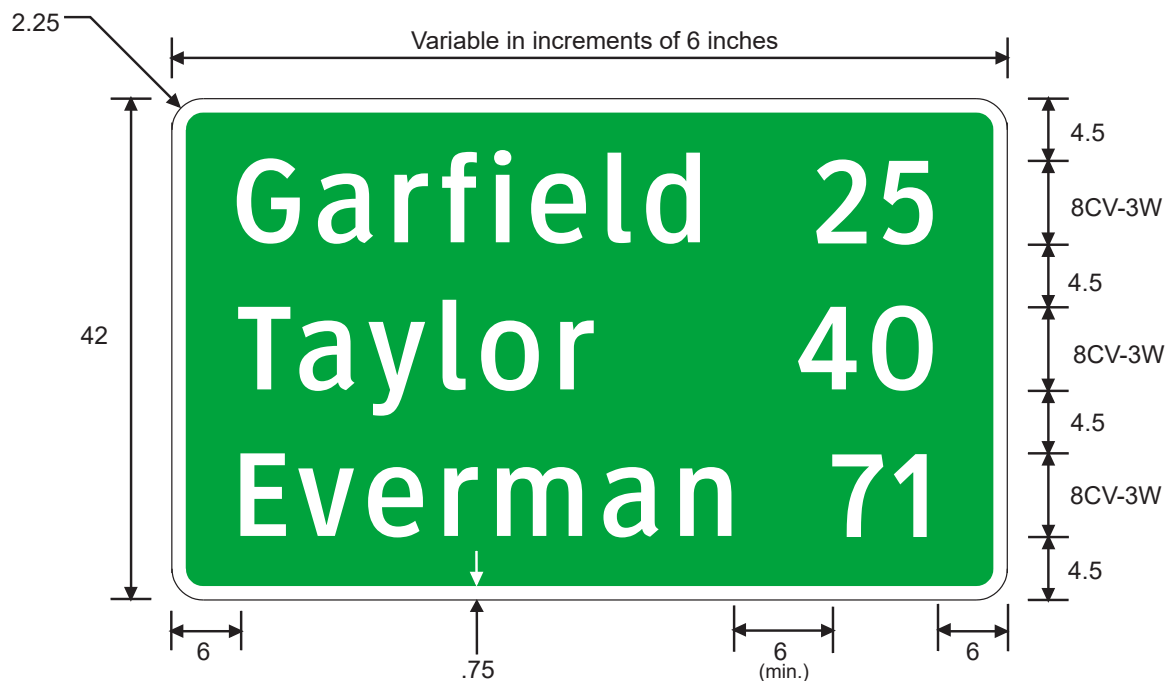
D2-3
