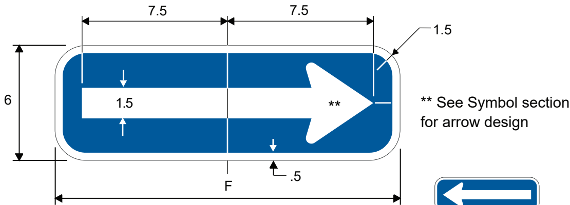
D5-5aTPR
