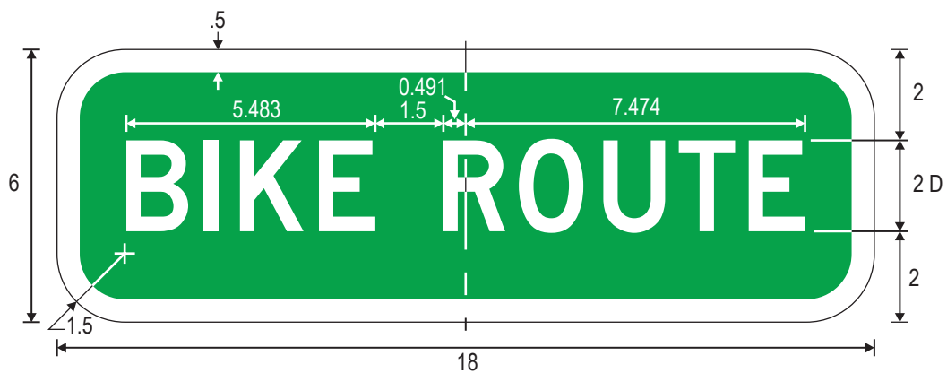
D11-1bP
