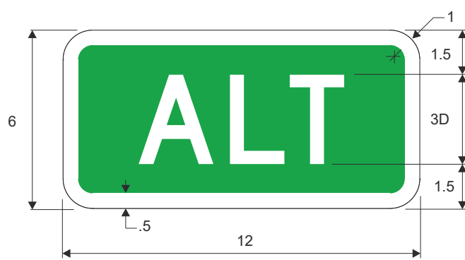
M4-1aG* ALT
