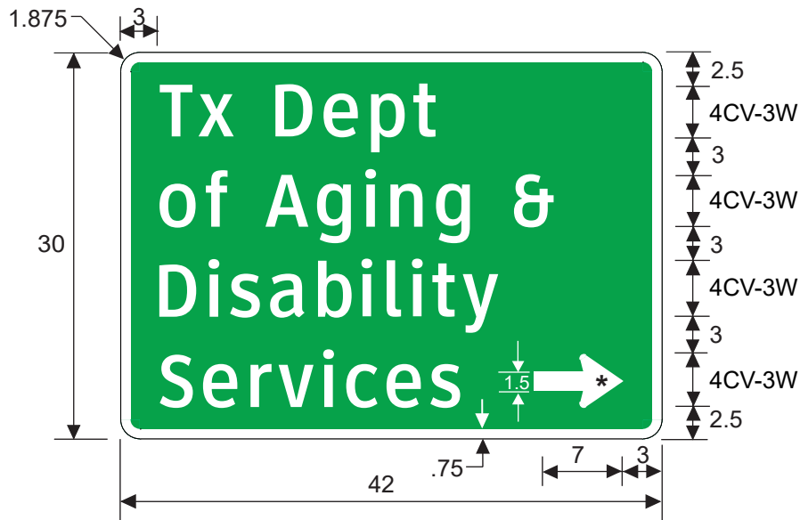
D26-4TR
