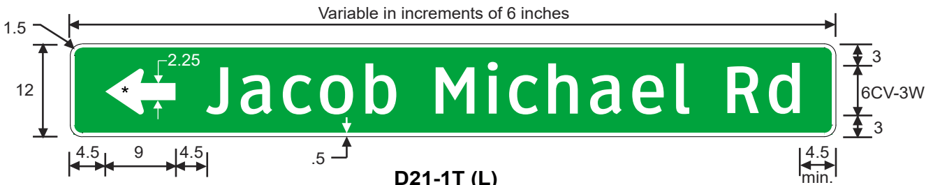
D21-1T (L)
