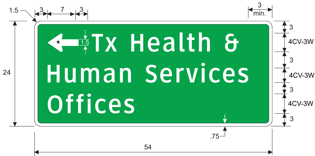
D26-7TL
