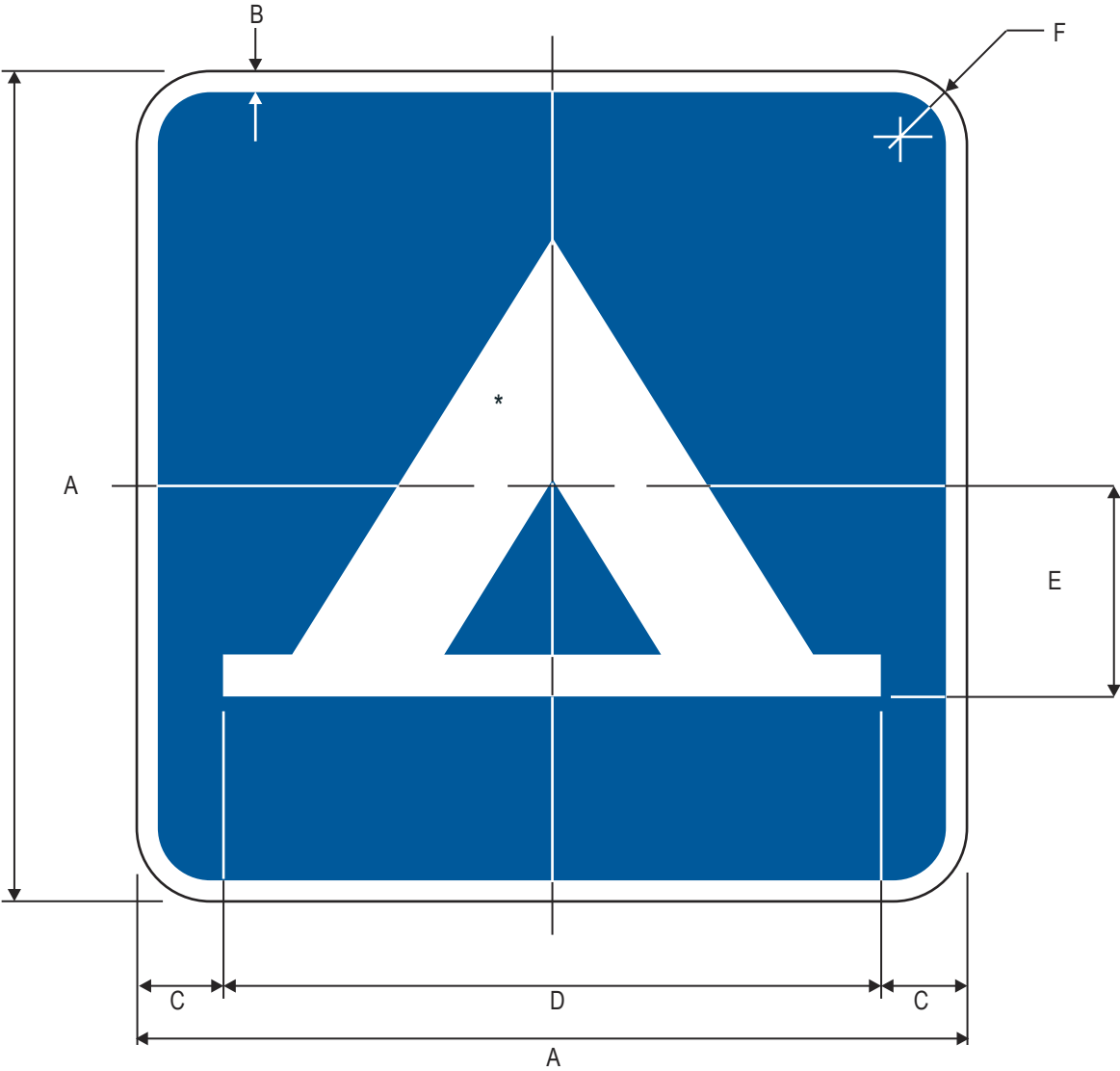
D9-3 Camping (Plaque)
