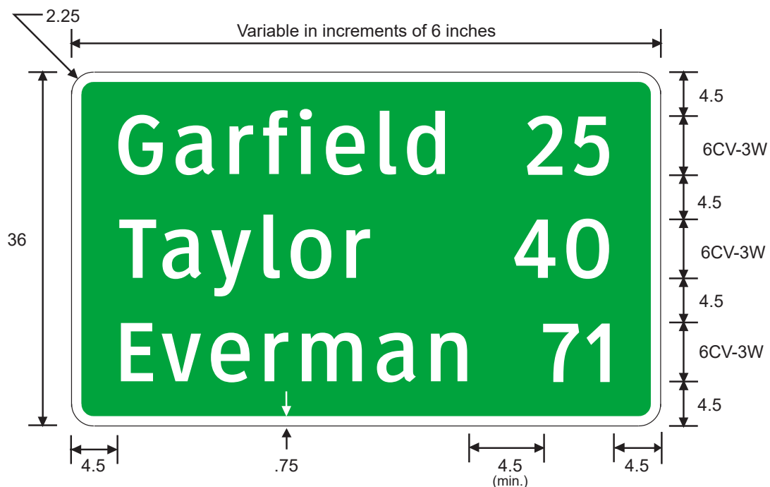
D2-3 Distance (3 line)
