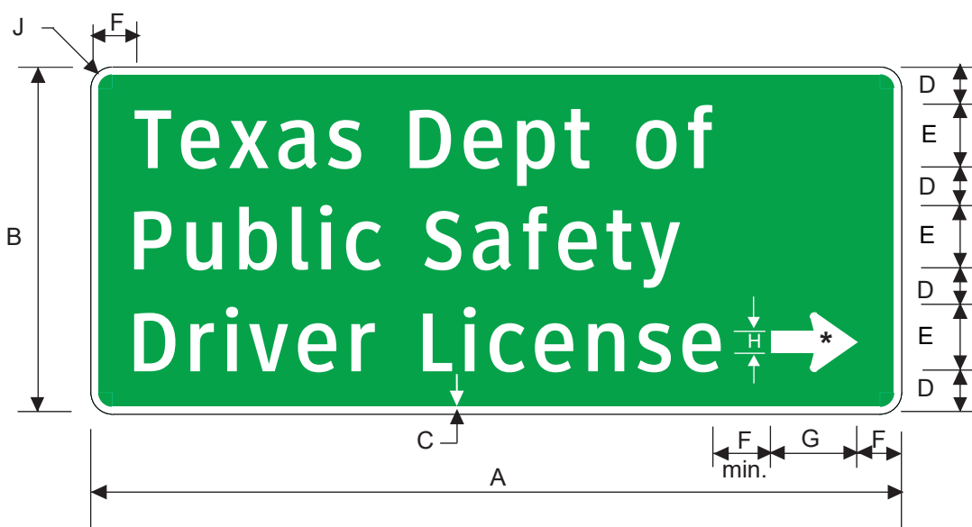
D26-2TR
