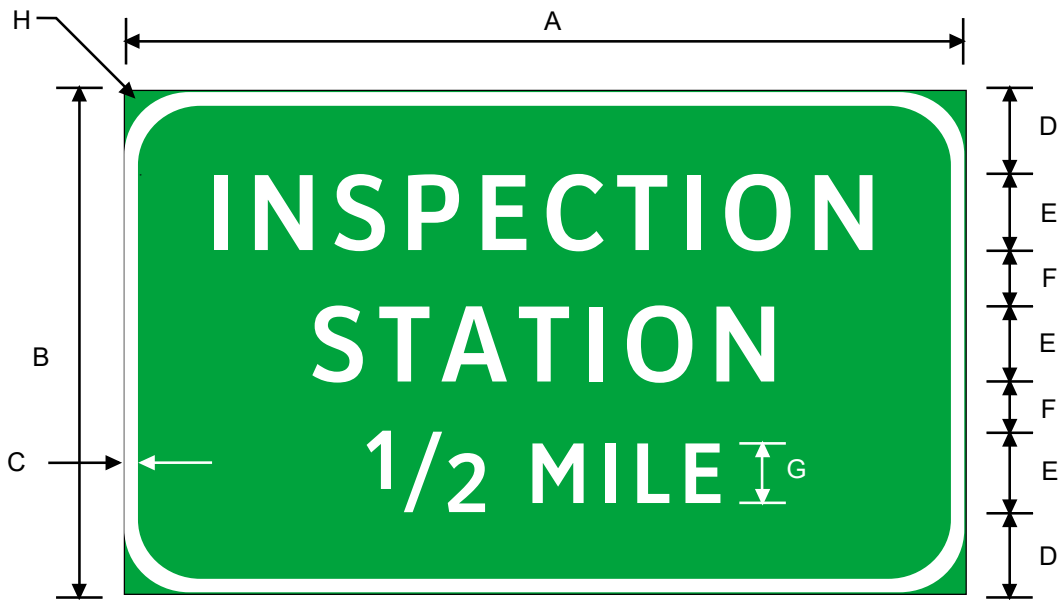
D8-2aT
