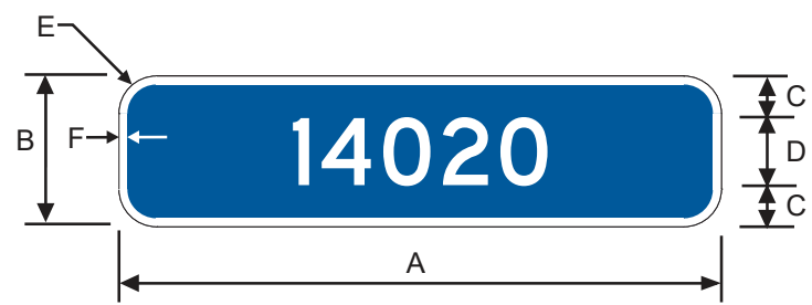
D5-2aTP
