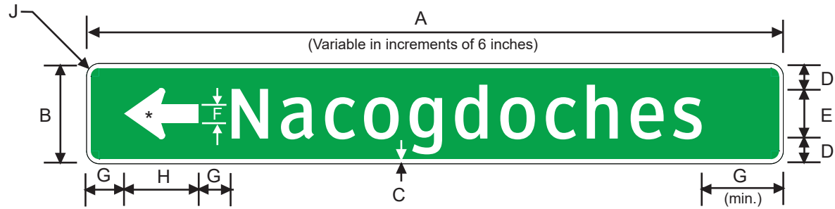
D1-1L
