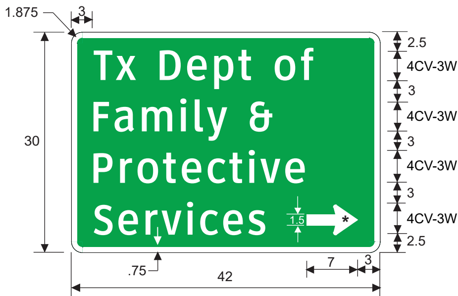
D26-5TR
