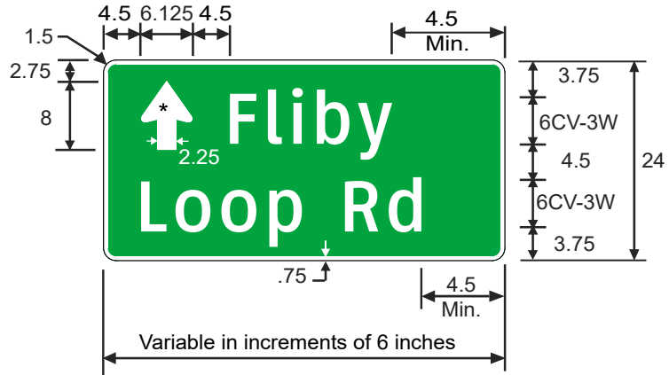
D21-1aT (UP)
