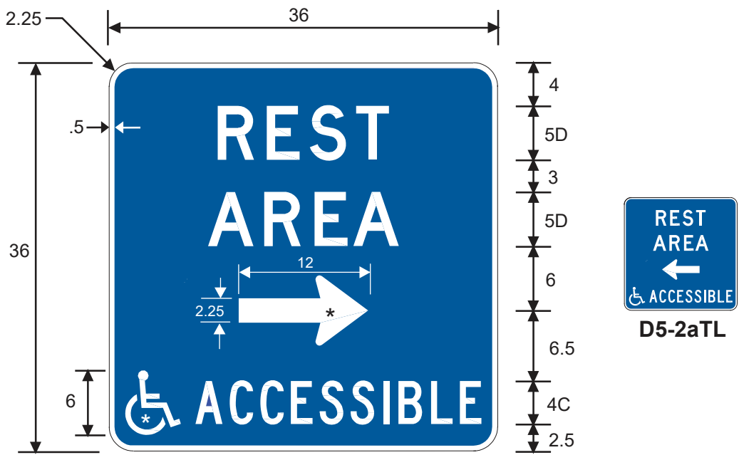
D5-2aTR
