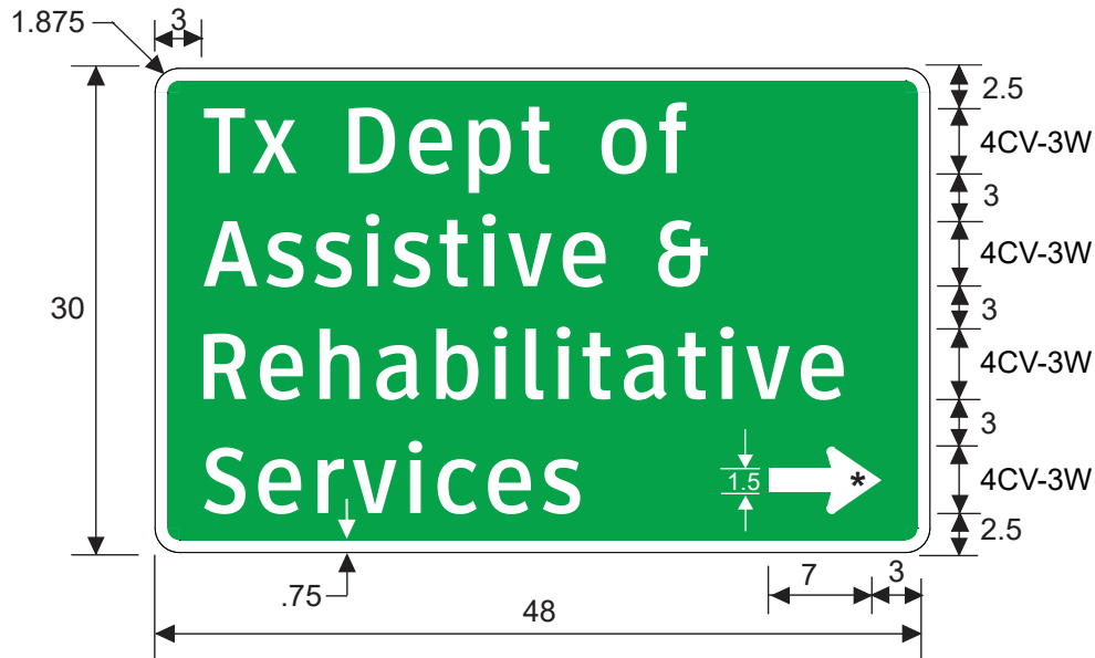
D26-6TR
