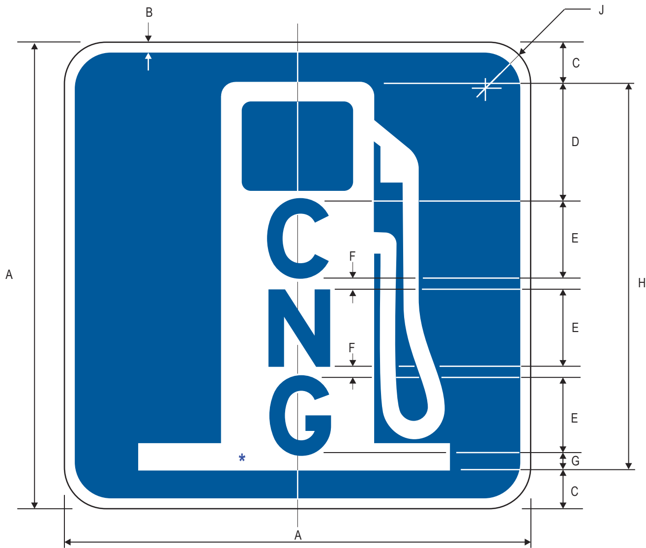
D9-11a
