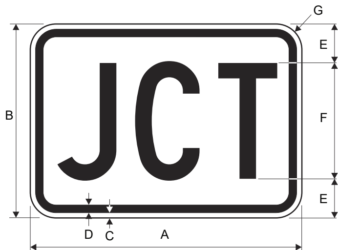
M2-1 JCT
