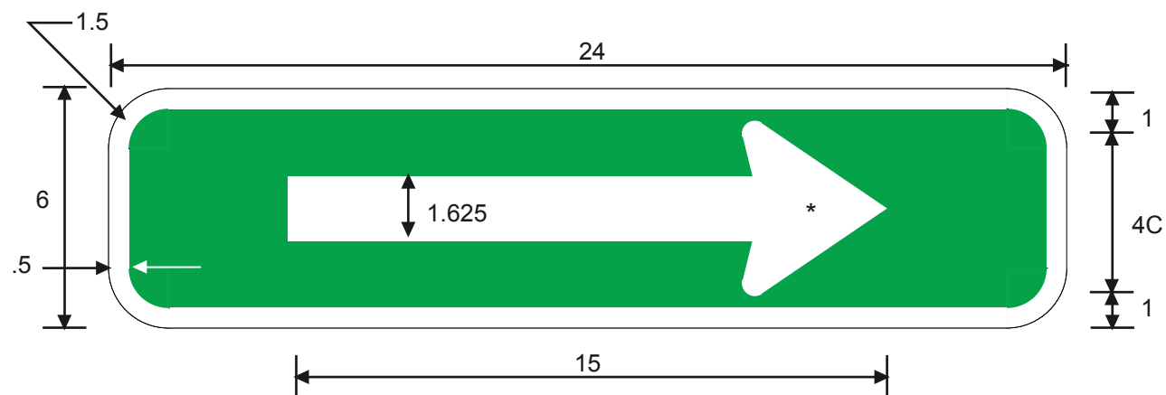
I-ARW
