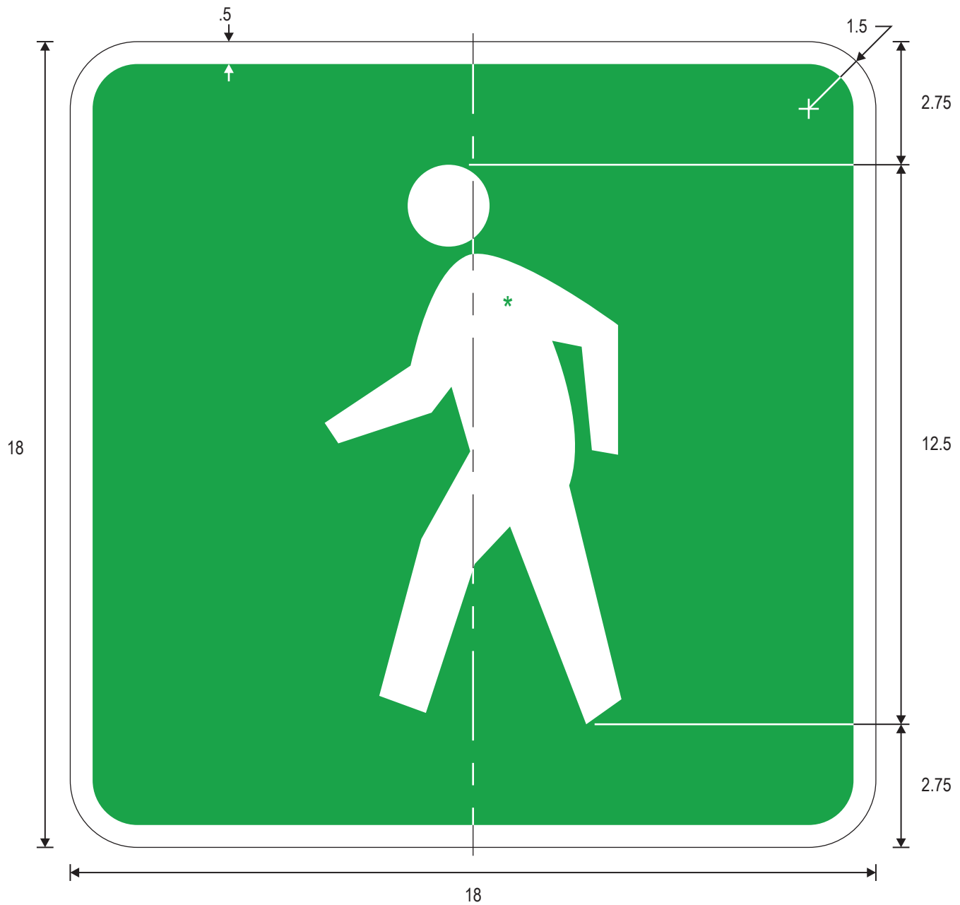
D11-2 Pedestrian (Symbol)
