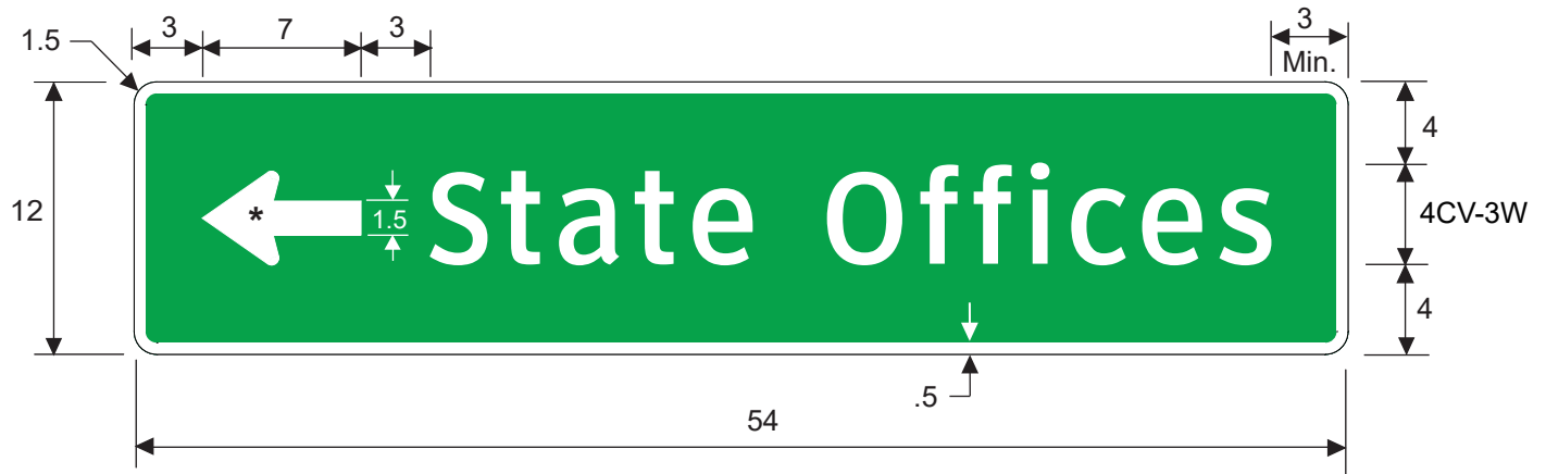
D26-8TL
