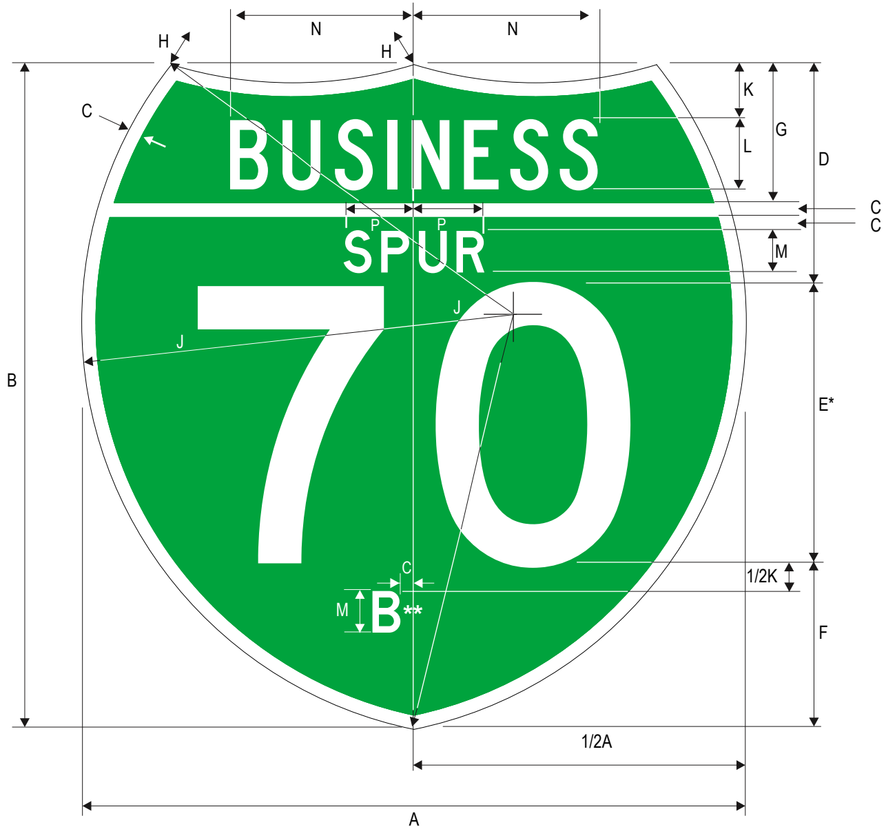
M1-3
