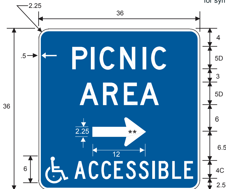
D5-2bTR
